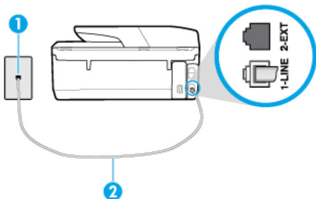
5-1. ábra: A nyomtató hátoldala
